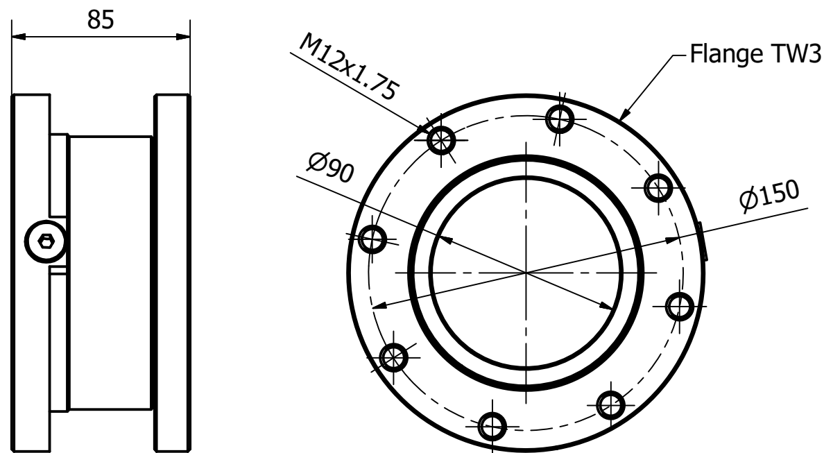
DN100 (4")
