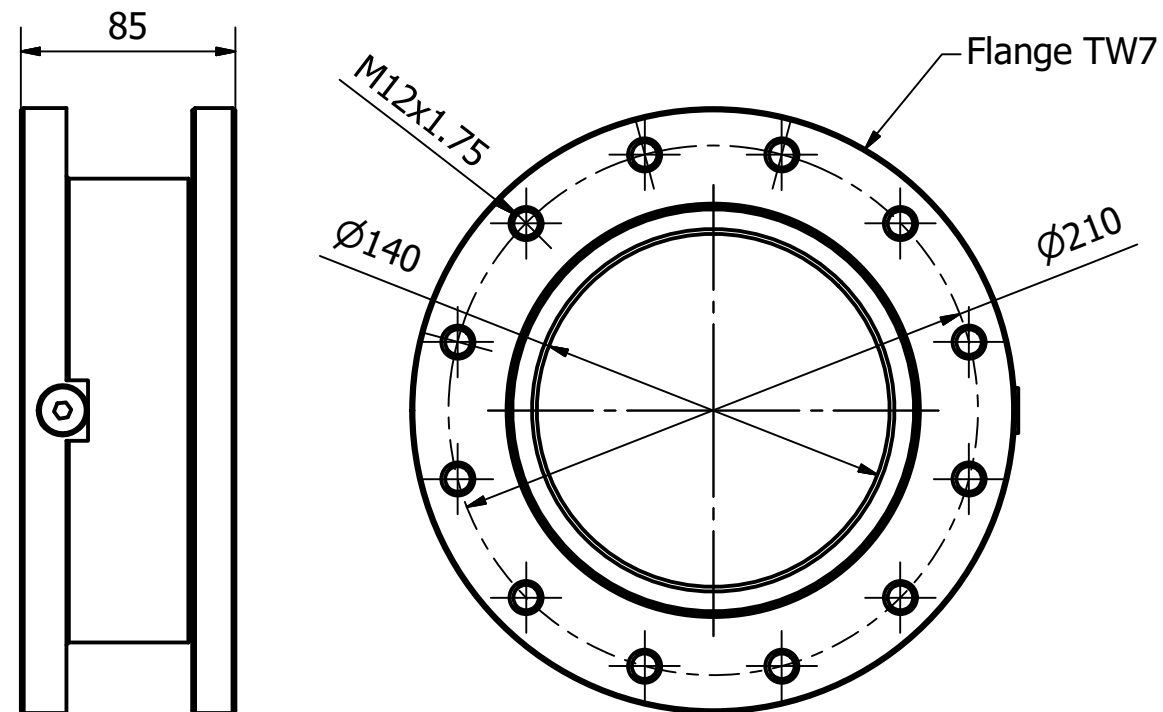
DN150 (6")
